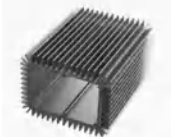
DA-CDAA-KHVL1 Tr.lượng/Weight: 6.423 kg/m Độ dày/Thickness: 2.0 mm
