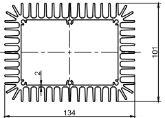
DA-CDAA-KHVL1 Tr.lượng/Weight: 6.423 kg/m Độ dày/Thickness: 2.0 mm
